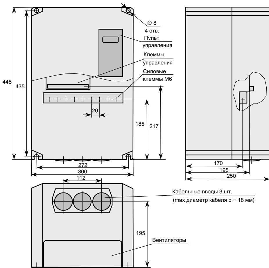
Масса 16 кг
